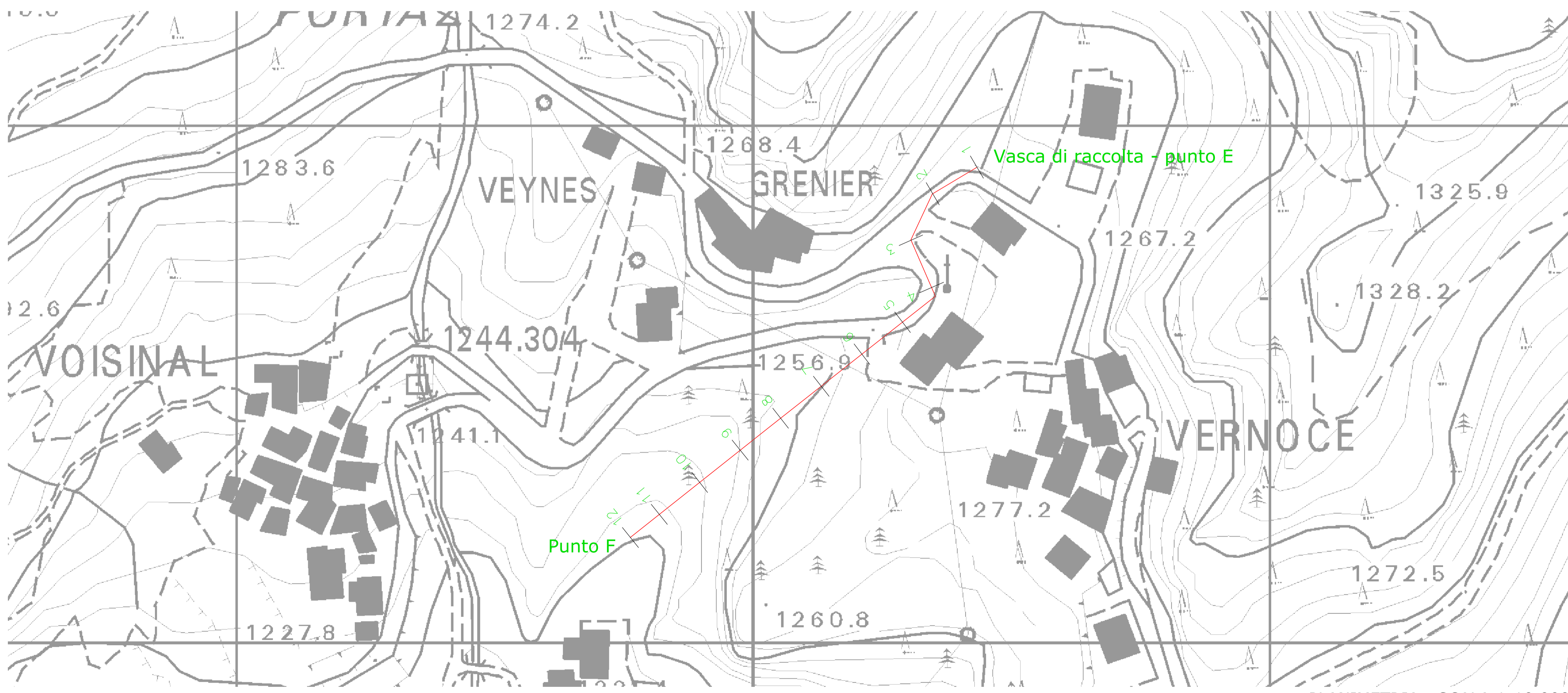
PLANIMETRIA - SCALA 1:10.000
